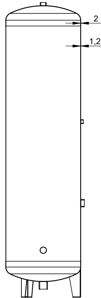
SECTION A-A
