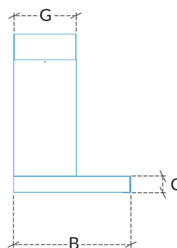
Seitenansicht
