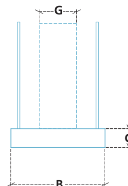
Seitenansicht
