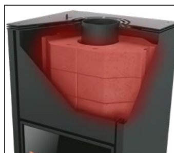
Wärmespeicher-System (nur für Serie X Plus)
