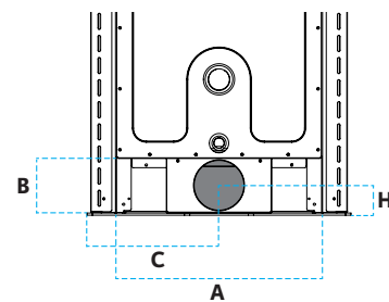
Hinteransicht
