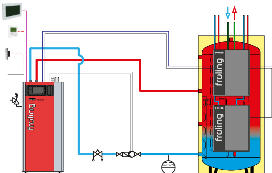
P5 Pellet mit Modulschichtspeicher HS, Frischwasserstation FWS und Heizkreisstation HKS
