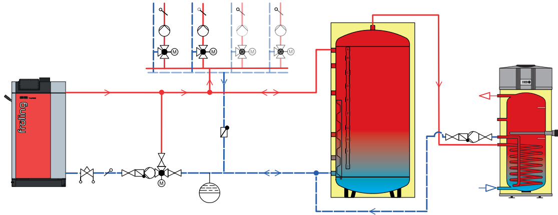
S2 Turbo mit Schichtspeicher und Brauchwasserwärmepumpe
