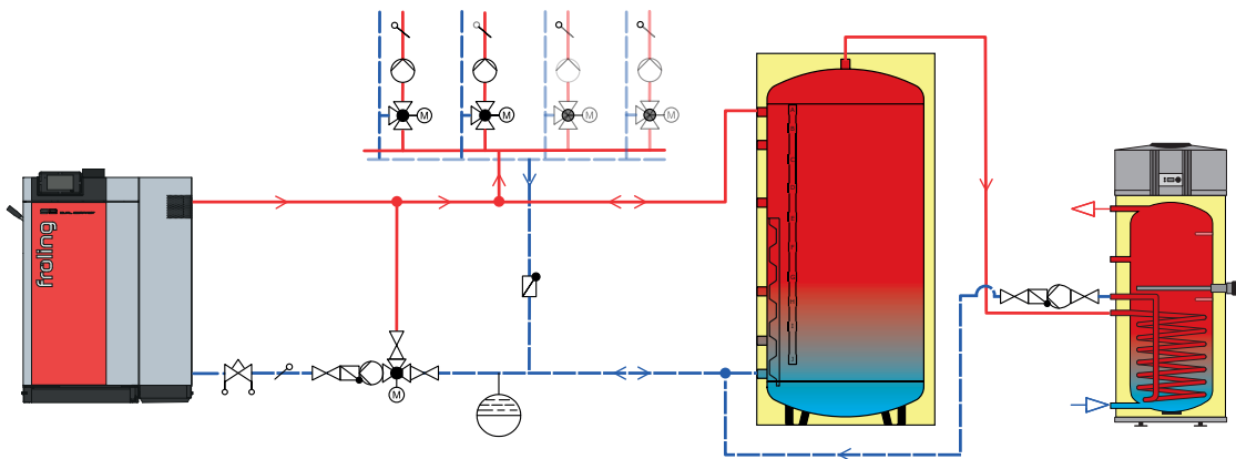
S5 Dual mit Schichtspeicher und Brauchwasserwärmepumpe
