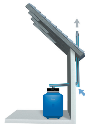
Raumluftunabhängige Aufstellvariante mit Rohr-in-Rohr-Kunststoff-Abgassystem entlang der Außenfassade.
