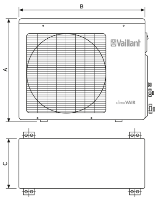
Außeneinheit
